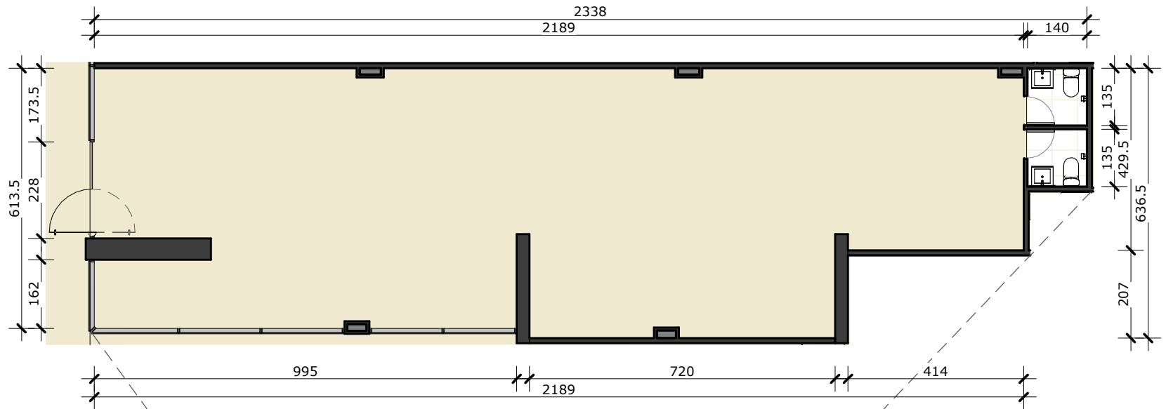
PLANTA LOCAL 100
